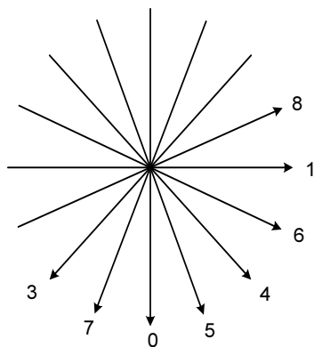
图 8-1—Intra_4x4各预测模式的方向（资料性）
